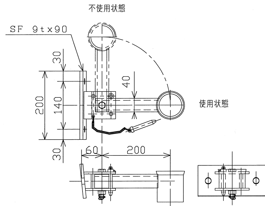
A-A矢視図
