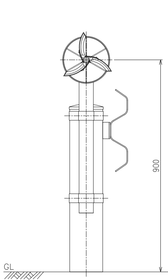
設置図 S=1:10
