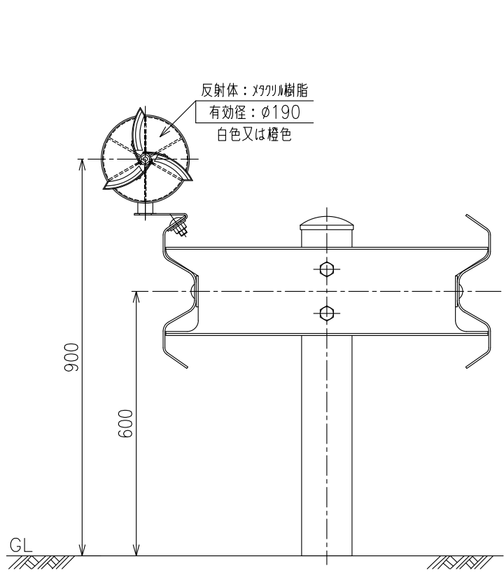
設置図 S=1:12
